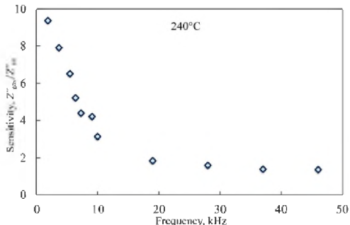
Նկ. 15 ZnO+1ատ.\%La սենսորի զգայունության կախվածությունը հաճախությունից՝ որոշված իմպեդանսային սպեկտրոսկոպիայի մեթոդով:
