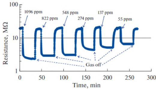
Սկ. 7 Fe_2O_3:ZnO սենսորի դիմադրության փոփոխությունն ամոնիակի գոլորշիների փարբեր կոնցենտրացիաների նկատմամբ 250°C աշխատանքային ջերմաստիճանում:
