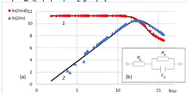
Նկ. 19 200°C ջերմաստիճանում Fe_2O_3:ZnO սենտորի իմպեդանսի իրական (1) և կեղծ (2) բաղադրիչների փորձարարական (կետեր) և տեսական մեթոդներով հաշվարկված (գծեր) արժեքների հաճախային կախվածությունները (a) և զգայուն կառուցվածքի համար առաջարկված համարժեք էլեկտրական շղթան (b) :
