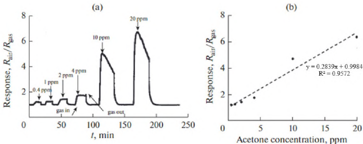
Սկ. 8 Fe_2O_3/SnO_2 սենսորի արձագանքը ացետոնի գոլորշու փարբեր կոնցենտրացիաների դեպքում (400 ppb- 20 ppm) (a) և սենսորի արձագանքի կախվածությունը ացետոնի գոլորշու կոնցենտրացիայից (b):
