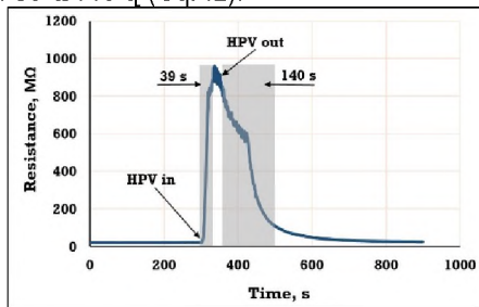
Նկ. 12 SnO 2 :PU (75:25 կշռ. %) սենսորի դիմադրության փոփոխությունը՝ ՋՊԳ-ի 3 ppm կոնցենտրացիայի դեպքում:
