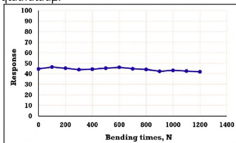
Նկ. 13 SnO 2 :PU (75:25 կշռ.%) ճկուն սենսորի արձագանքի սենսորի բազմակի ճկումների դեպքում:
