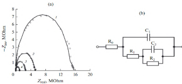
Նկ. 18 ԲԱՆԽ/SnO 2 սենսորի Նայքվիստի կորերը (օդ (1), 4 ppm (2), 10 ppm (3), 20 ppm (4)) 250°C աշխատանքային ջերմաստիճանում (a) և առաջարկվող համարժեք էլեկտրական շղթան (b):
