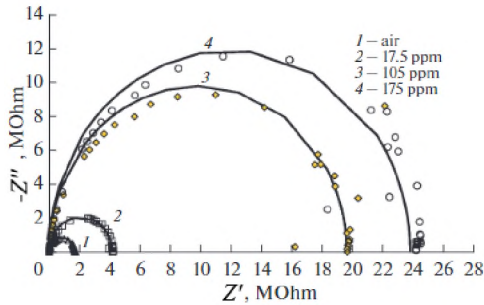
Նկ. 17 ZnO+2ադ. % La թաղանթի Նայքվիստի կորերը, ՋՊԳ-ի փարբեր կոնցենտրացիաների դեպքում՝ 175°C աշխատանքային ջերմաստիճանում: Կետերը ներկայացնում են փորձարարական տվյալները, հոծ գծերը՝ տեսական:
