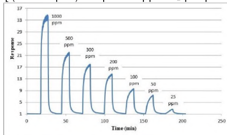
Նկ. 10 \text{FALiSnO}_2 (5:95 կշռ. %) ճկուն սենսորի արձագանքը ջրածնի փարբեր կոնցենտրացիաների նկատմամբ՝ 100°C աշխատանքային ջերմաստիճանում:
