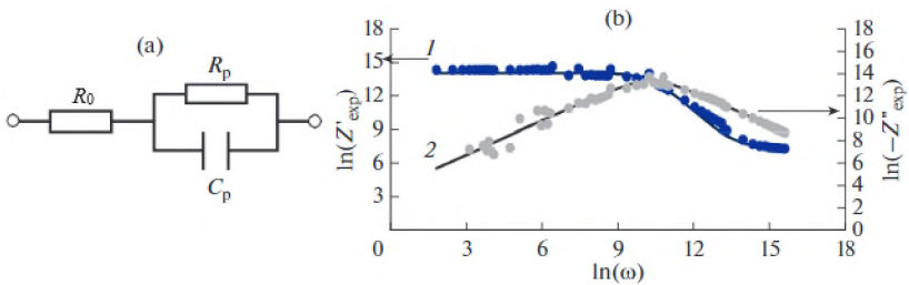
Նկ. 16 ZnO+2ատ.% La սենտորային կառուցվածքի համար առաջարկվող համարժեք էլեկտրական շղթան (a) և 200°C ջերմաստիճանում փորձարարական (կետեր) և տեսականորեն հաշվարկված (հոծ գծեր) հաճախային կախվածությունները՝ իմպեդանսի իրական և կեղծ մասերի համար (b):
