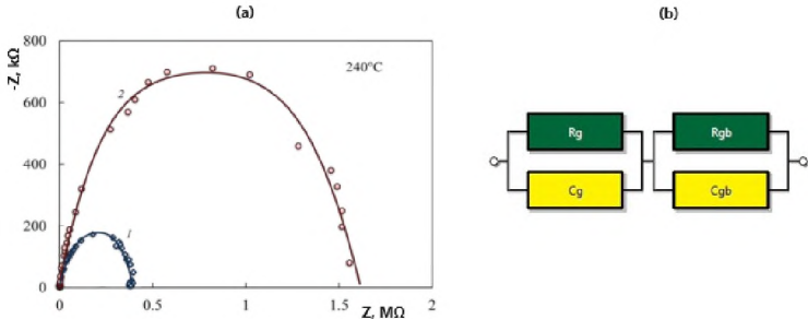
Նկ. 14 ZnO+1ատ.\%La սենսորի Նայքվիստի դիագրամը օդում (1) և ՋՊԳ-ի ազդեցությամբ (2) (a) ու սենսորի համար ընտրված համարժեք էլեկտրական շղթան (b):
