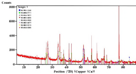
Նկ. 5 SnO 2 :PULSU (75:25 կշռ.%) թաղանթի ռենտգենյան պատկերը:
