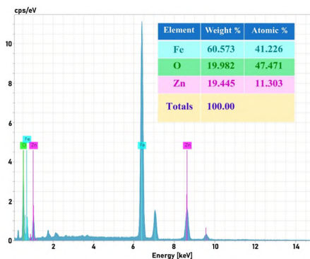
Նկ. 4 Fe_2O_3:ZnO (80:20 կշն.%) թաղանթի փարրային անալիզի (EDX) արդյունքները:
