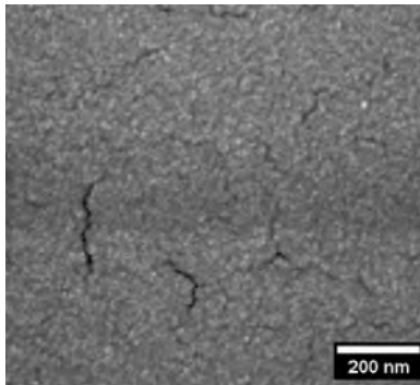
Նկ. 3 Fe_2O_3:ZnO (80:20 կշն.%) թաղանթի ՏԷՄ պատկերը:
